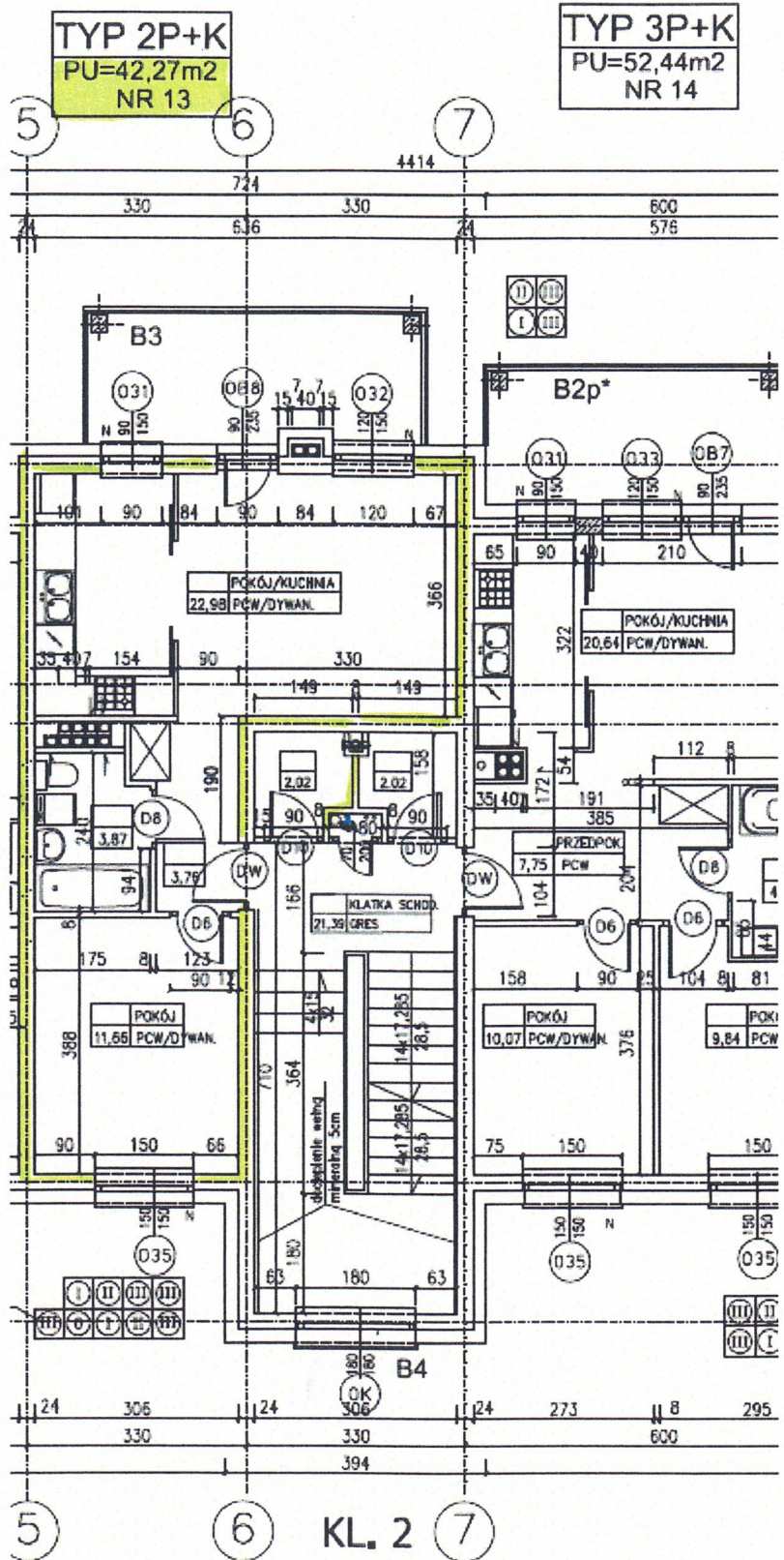
RZUT III PIĘTRA BUDYNEK NR 4
